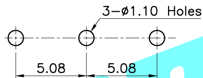
P.C.B layout
